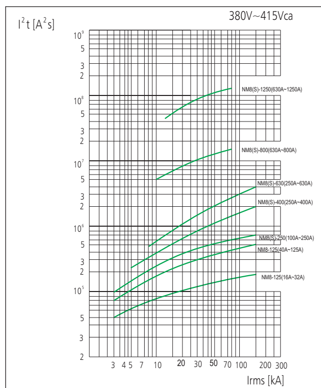
A^2s curva
