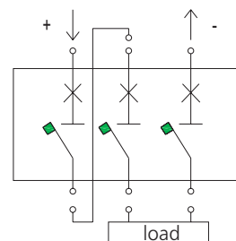
Esquema B: Interrupción con dos polos en serie para una polaridad y un polo para la otra polaridad.
